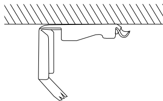
figuur 1b: plafondbevestiging
